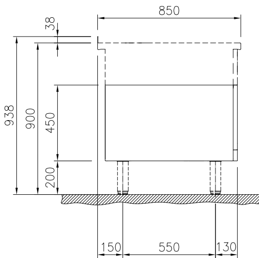
俯视
